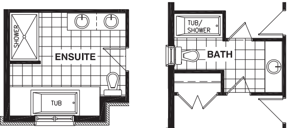
OPTIONAL 5PC ENSUITE OPTIONAL JACK & JILL
